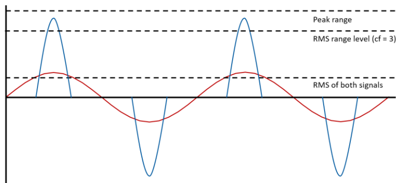
Abb.3: Vergleich zweier Signale mit gleichem Effektivwert und unterschiedlichen Scheitelfaktoren
